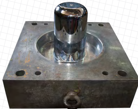
JUG PUNCH MOULD
