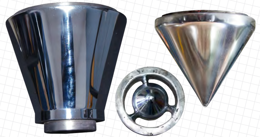
SPIDER PVC PIPE DIE HEADS
